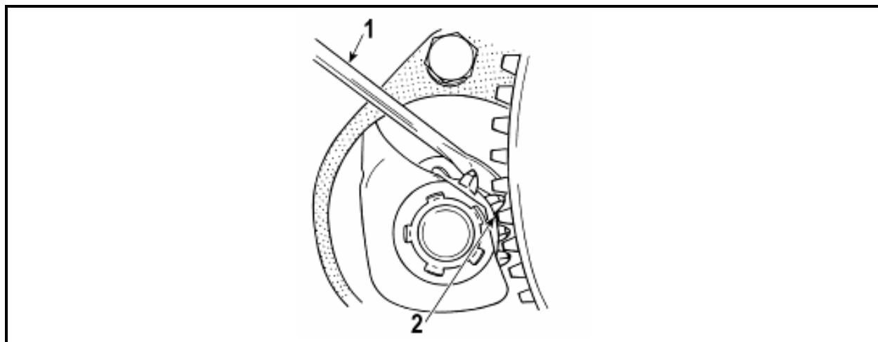
Рисунок 40 – Проверка зазора между зубьями
